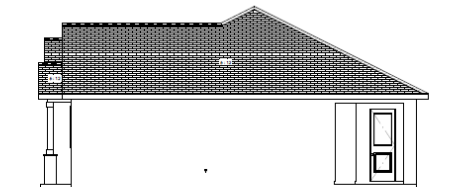
RIGHT ELEVATION
